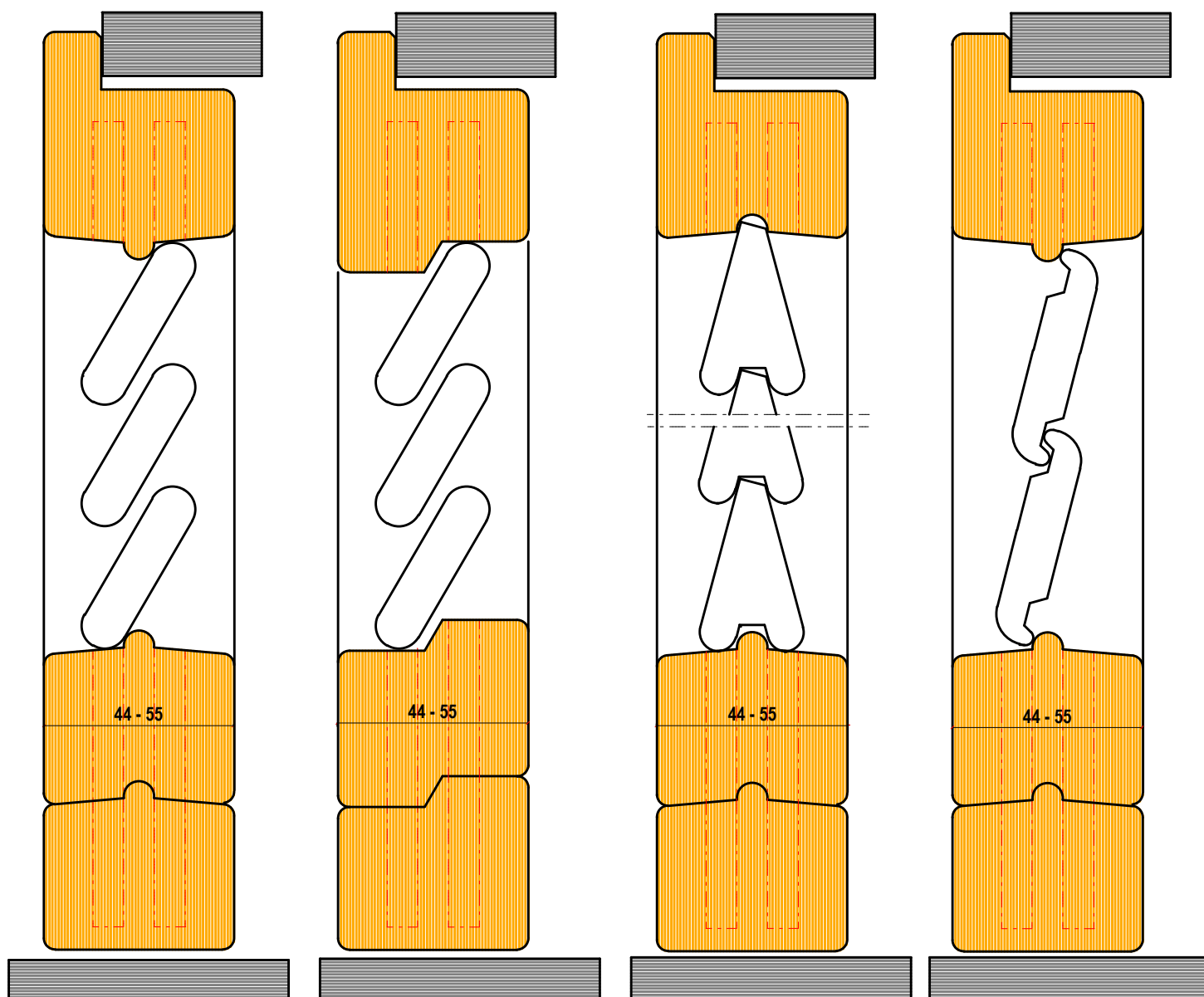
SEZIONE VERTICALE
