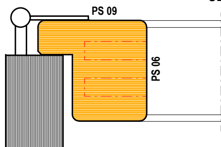
SEZIONE VERTICALE
