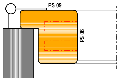
SEZIONE VERTICALE
