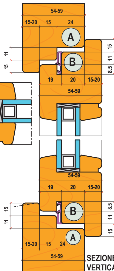
ESEMPIO DI FINESTRA SENZA TENONI WINDOW WITHOUT TENONS
