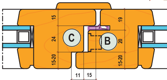
VARIANTE PORTA CON ALLUMINIO
