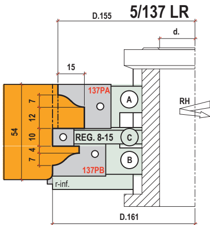
TENONE SEMPLICE CON RAGGI SPESSORE 54-59 mm THICKNESS 54-59mm
