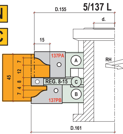
TENONE SEMPLICE SPESSORE 45-54 mm THICKNESS 45-54 mm
