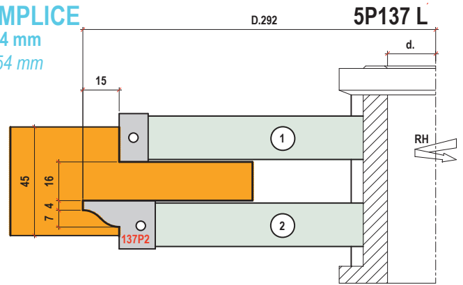
TENONE SEMPLICE CON RAGGI SPESSORE 54-59 mm THICKNESS 54-59mm
