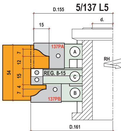
TENONE DOPPIO SPESSORE 54-56 mm THICKNESS 54-56 mm
