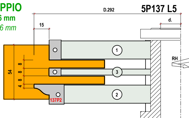
5/137 L5R TENONE DOPPIO CON RAGGI SPESSORE 54-59 mm THICKNESS 54-59 mm
