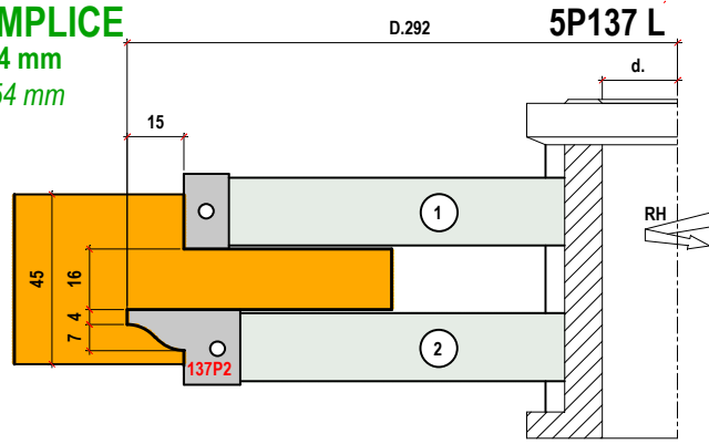
5/137 LR TENONE SEMPLICE CON RAGGI SPESSORE 54-59 mm THICKNESS 54-59mm
