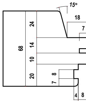
08 TRAVERSO INF TELAIO
