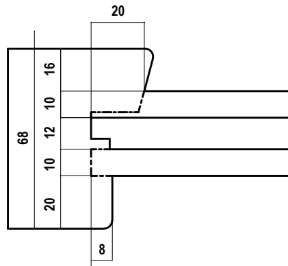
05 FEMMINA TELAIO INF
