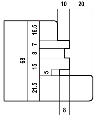
12 CHIUSURA CENTRALE SX
