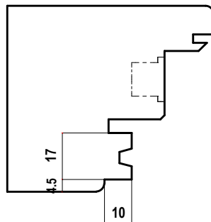
09 R RIPASSO ESTERNO ANTA
