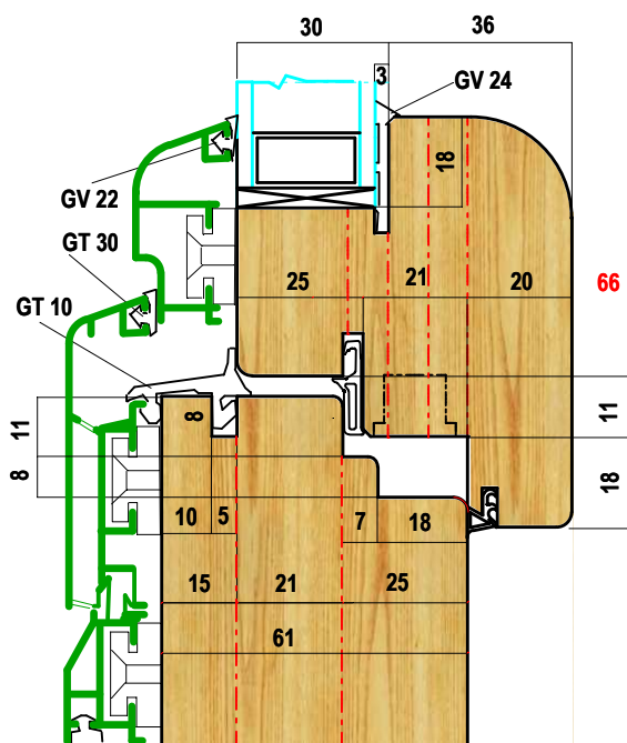
SEZIONE VERTICALE
