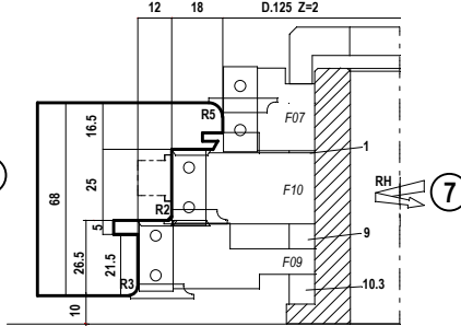
SQUADRATURA ANTA SQUARING SASH
