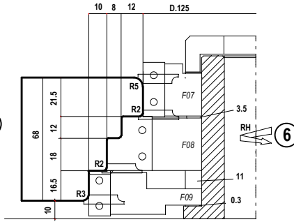
PROFILATURA MONTANTE CENTRALE ANTA SINISTRA PROFILING CENTRAL JAMB LEFT SASH
