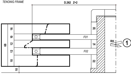
TENONATURA TELAIO TENONIG FRAME
