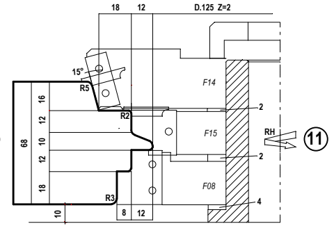
PROFILATURA TRAVERSO INFERIORE TELAIO PROFILING LOWER CROSS FRAME
