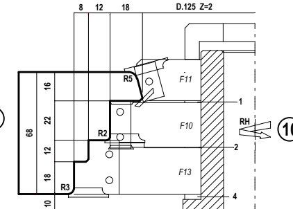
PROFILATURA TRAVERSO SUP. E MONTANTI TELAIO PROFILING FRAME CROSS AND JAMBS
