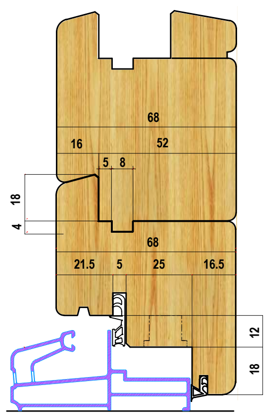
PORTA FINESTRA
