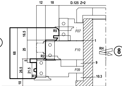
PROFILATURA INFERIORE ANTA PROFILING LOWER SASH
