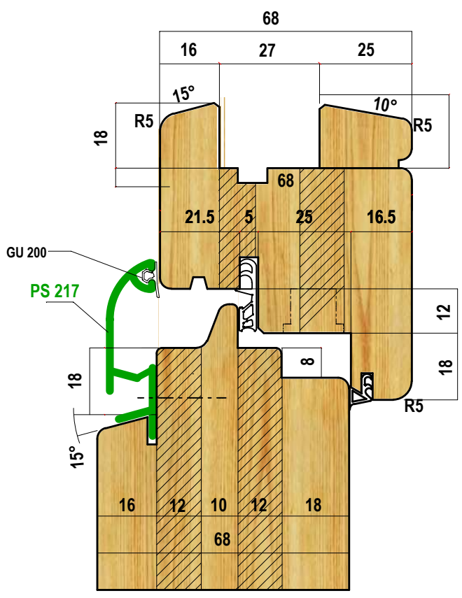
SEZIONE VERTICALE
