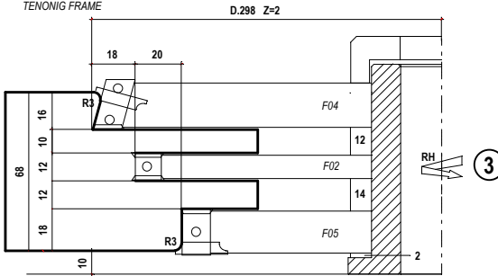
TENONATURA TELAIO TENONIG FRAME
