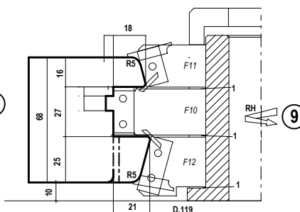
PROFILATURA INTERNO ANTA PROFILING INTERNAL SASH
